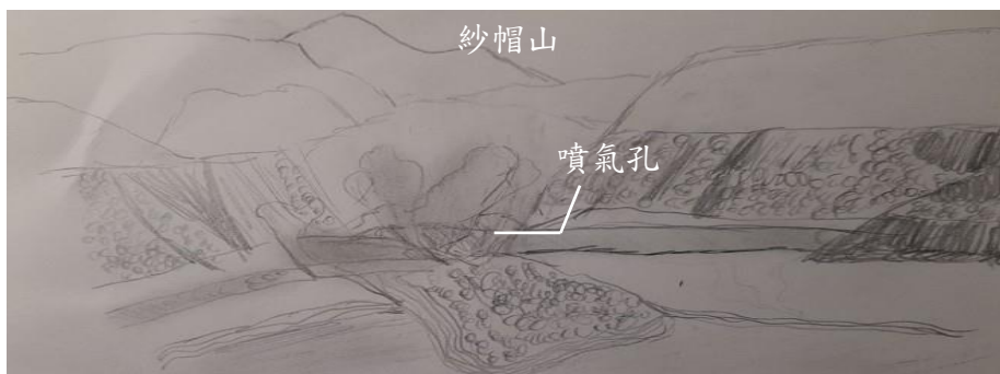
圖 3. 硫磺谷素描(自繪於硫磺谷，2024)
