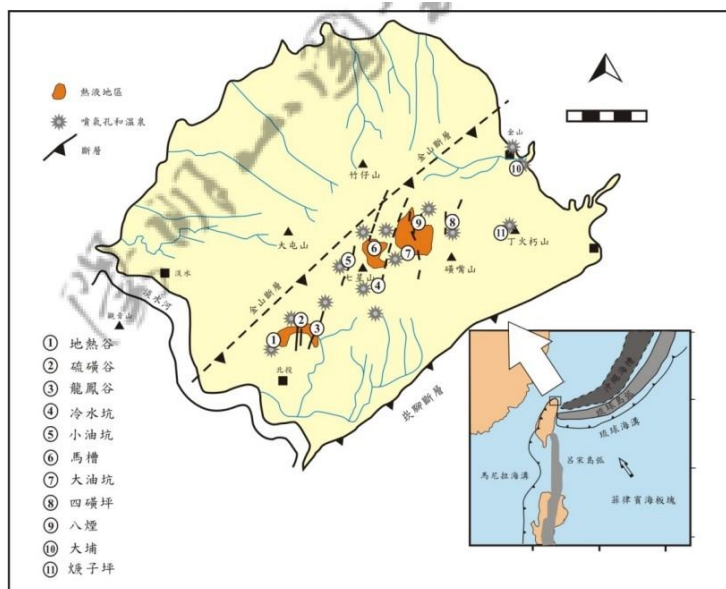
圖 6. 金山斷層(取自 https://www.moi.gov.tw/ ，2009)
